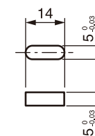
付属両丸平行キー
