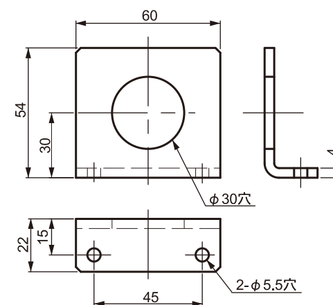
M30L (L型取付金具)
