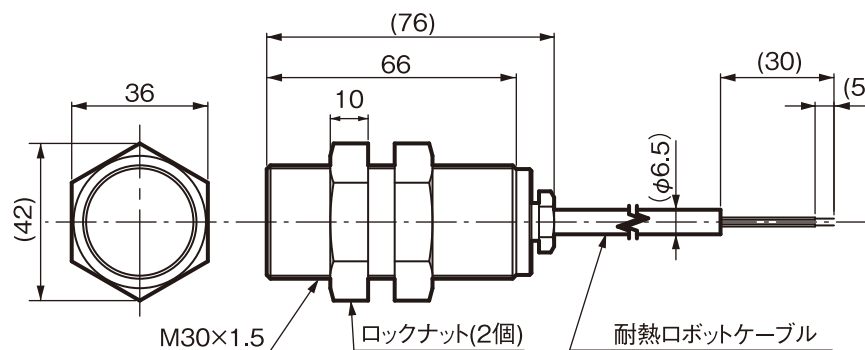
HPS-M30M (ネジ型センサ)
