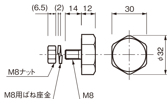
HPM-34(マグネット)
