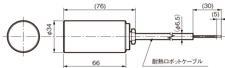
HPS-M34D (円筒型センサ)
