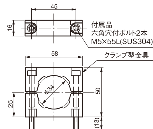
M34K (クランプ型取付金具)
