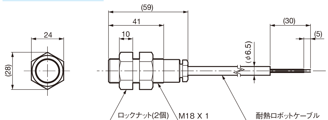
HPM-M18M (ネジ型センサ)
