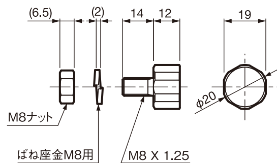
HPM-22 (マグネット)
