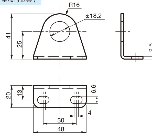
M18L(L 型取付金具)
